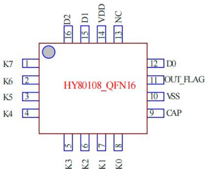
QFN16
