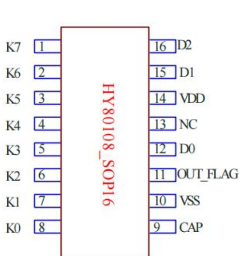
Sop16
